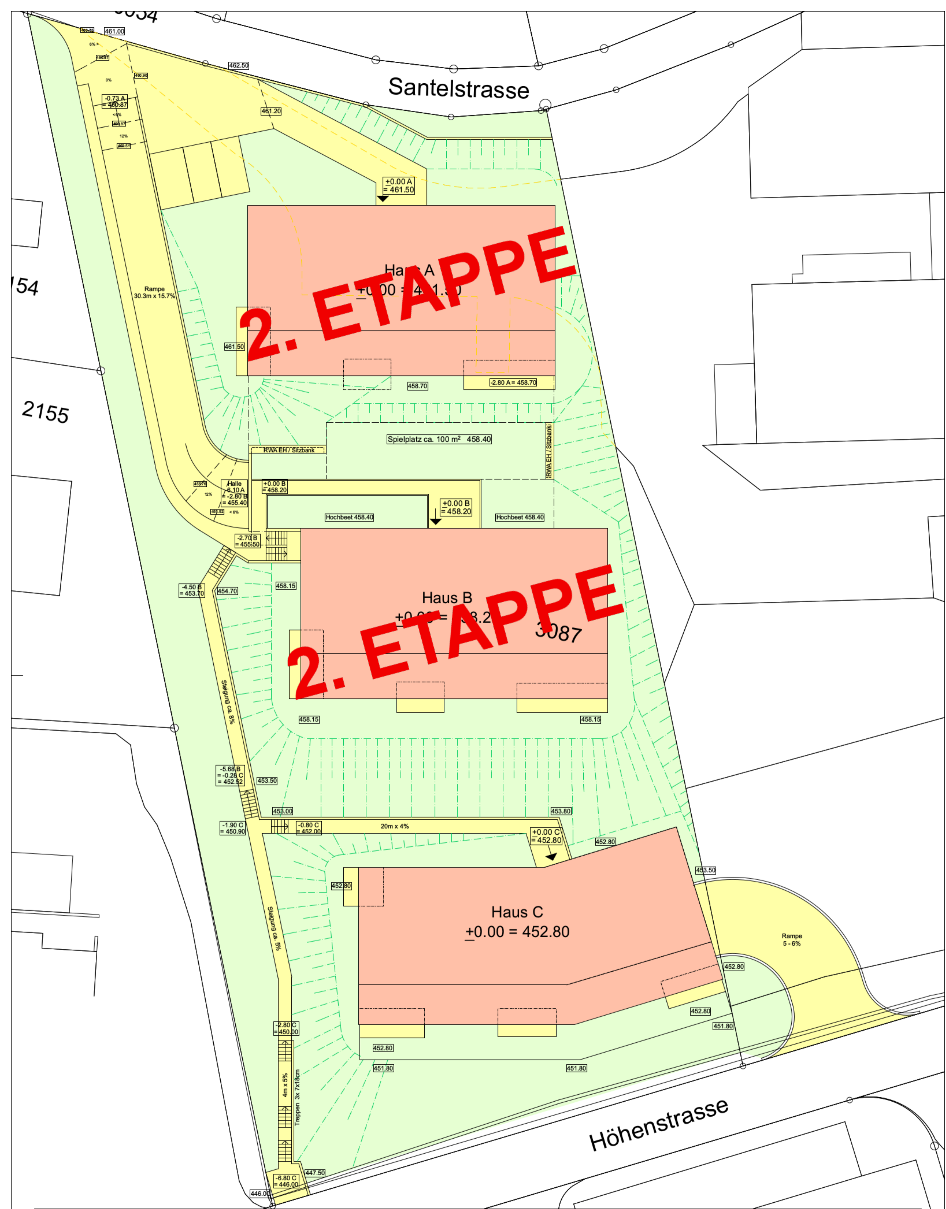
02 Umgebung 1:200
